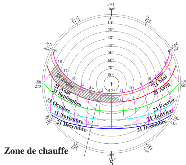
Figure A-1-19 : Diagramme solaire de Séradii
