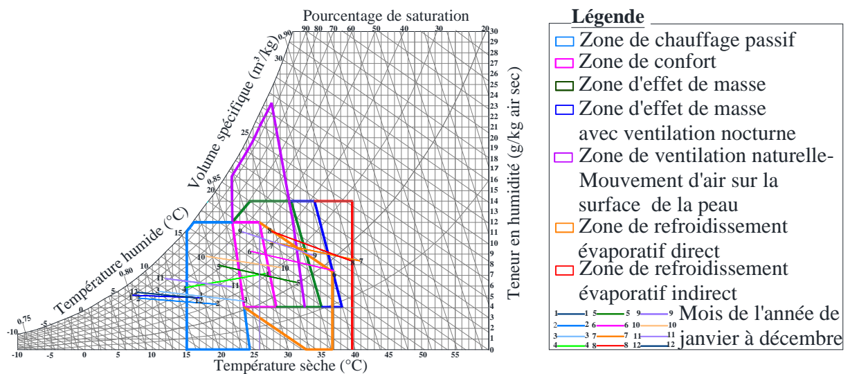
Figure II-10 : Diagramme psychrométrique de la région de Biskra
