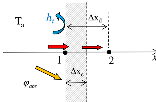
Figure III-3 : Discretisation spatiale des demi-tranches en surface
