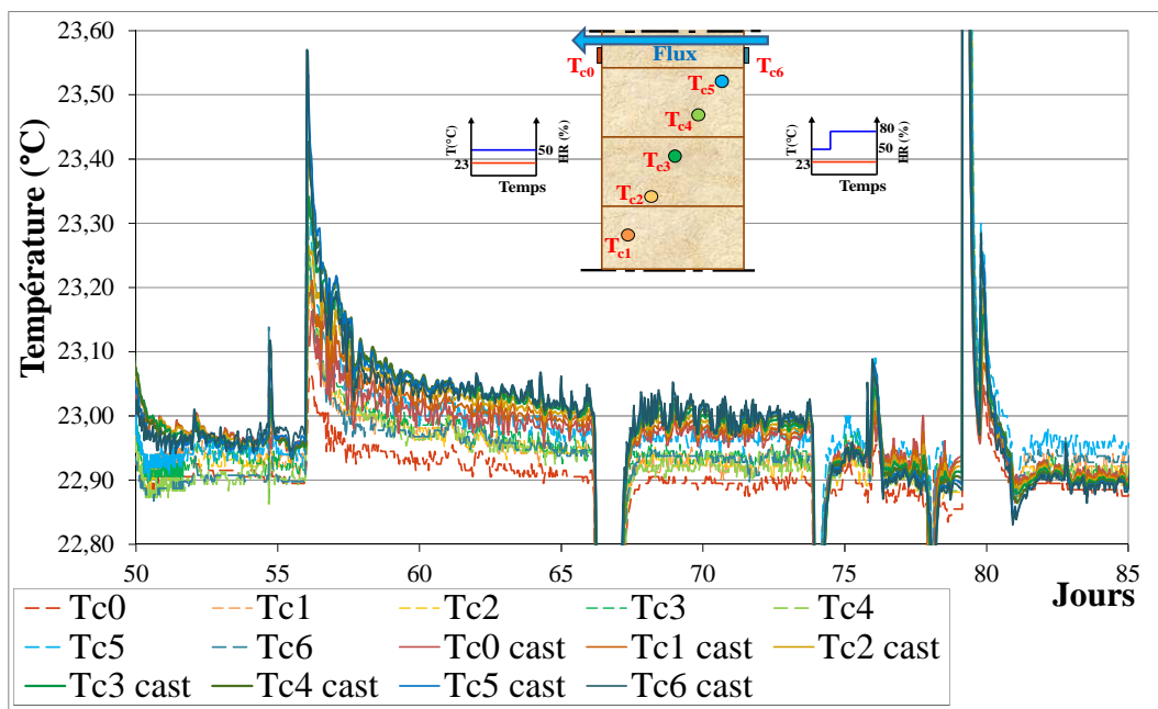
Figure V-23 : Profils thermiques mesurés et modélisés en phase d'adsorption
