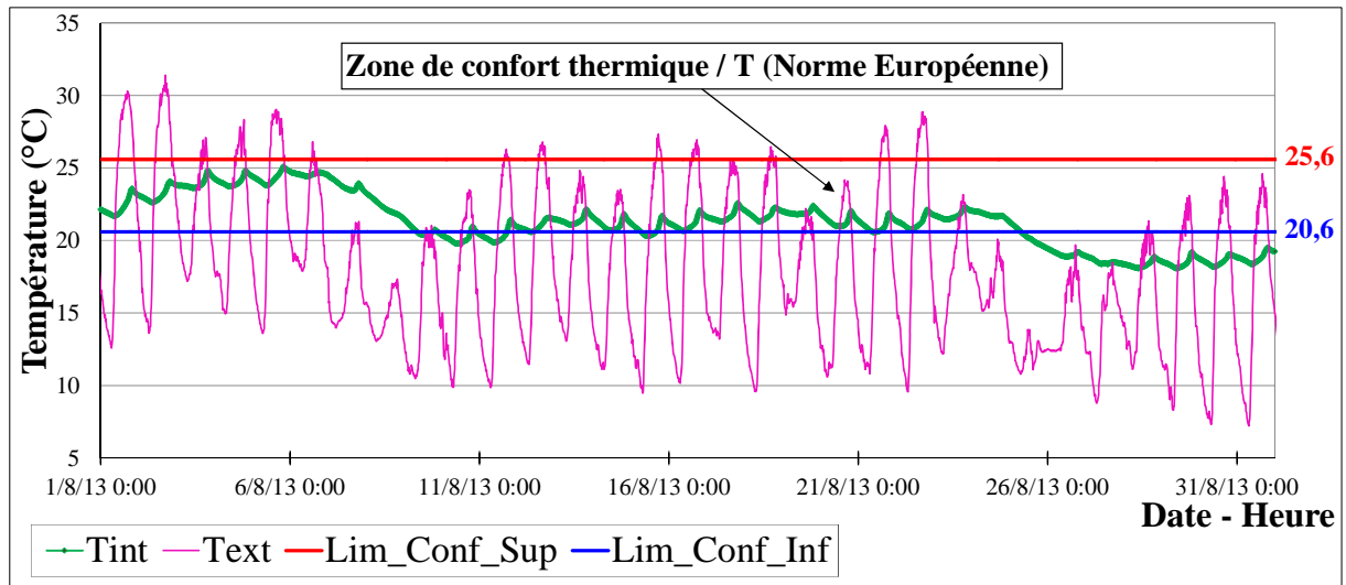
Figure C-4 : Températures et limites du confort thermique / T « fuste, mois d'août »
